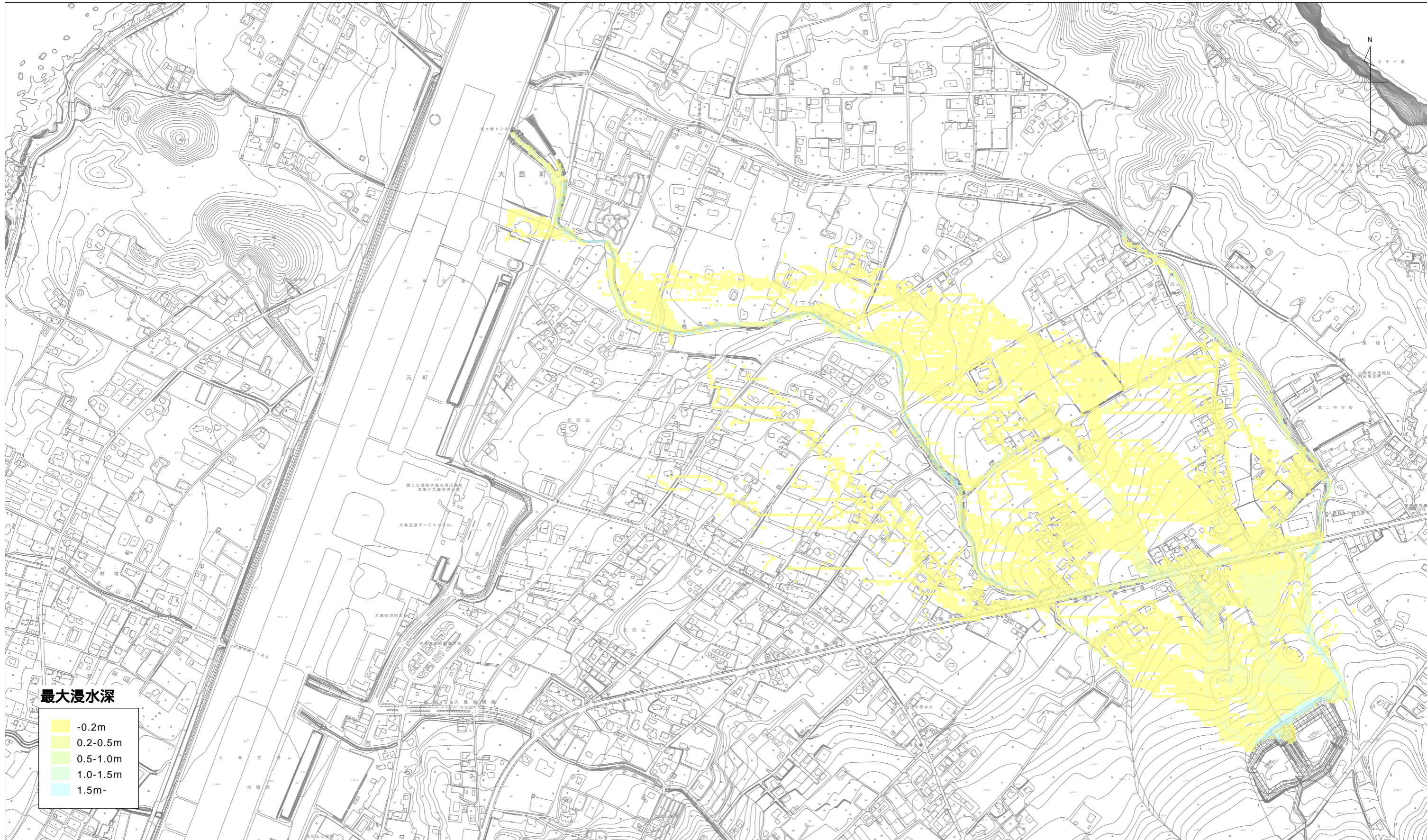
農業用ため池浸水想定区域図（沢立貯水池）
