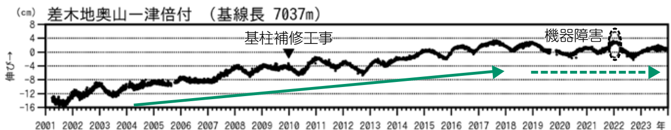
差木地奥山と津倍付のGNSS観測点間の距離変化のグラフ（2001年～2023年）
