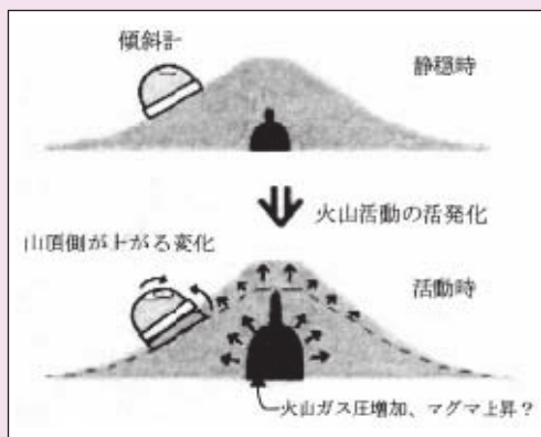
(図1) 地下のマグマ、ガスの動きと傾斜の変化
