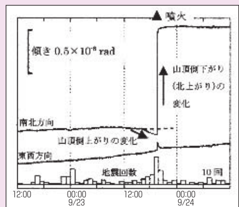
(図2) 浅間山の噴火前後の傾斜変化(2004年9月23日)
