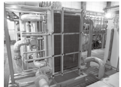
↑大島内燃力発電所 3号熱交換器
