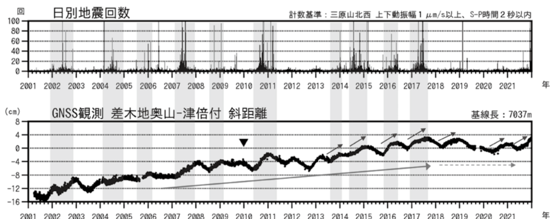
日別地震回数とGNSS観測点の距離変化のグラフ（平成13年～令和3年）
