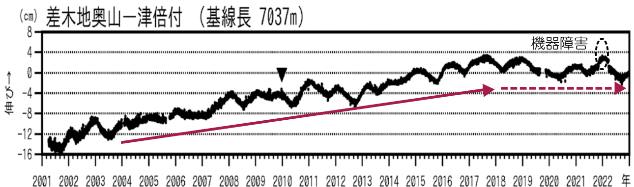
差木地奥山と津倍付のGNSS観測点間の距離変化のグラフ（平成13年～令和4年）
