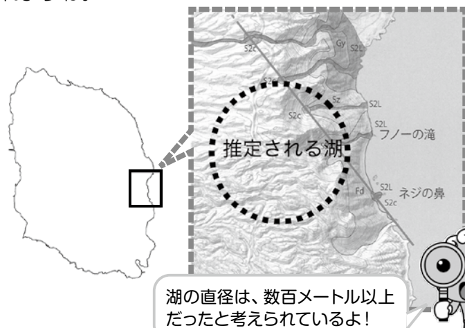
【図1：伊豆大島火山地質図（暫定版2022）】※1
