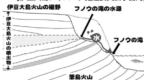
【図2：フノウの滝付近の東西断面図】※2
