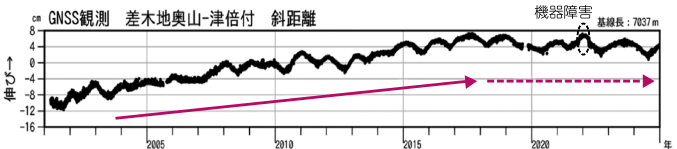
差木地奥山と津倍付のGNSS観測点間の距離変化（2001年～2024年）
