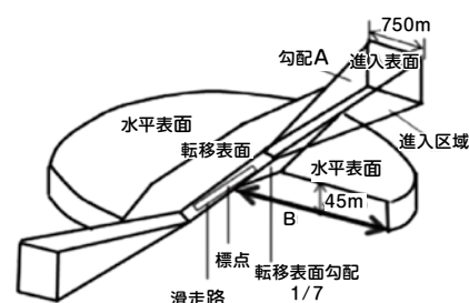
進入表面の勾配 (A) 大島空港 1/40
