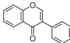
イソフラボン isoflavone C 15 H 10 O 2
