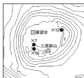
伊豆大島 火口底地表面最高温度(1991年5月～2005年6月)
