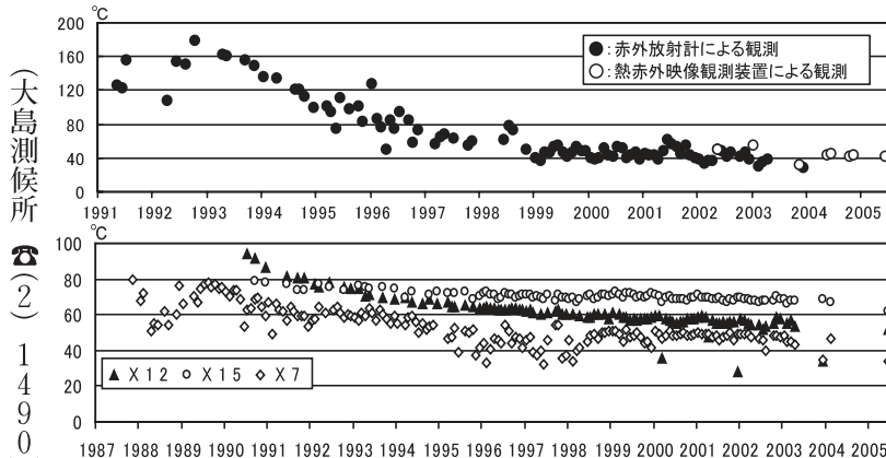
伊豆大島 火口底地表面最高温度(1991年5月～2005年6月)
