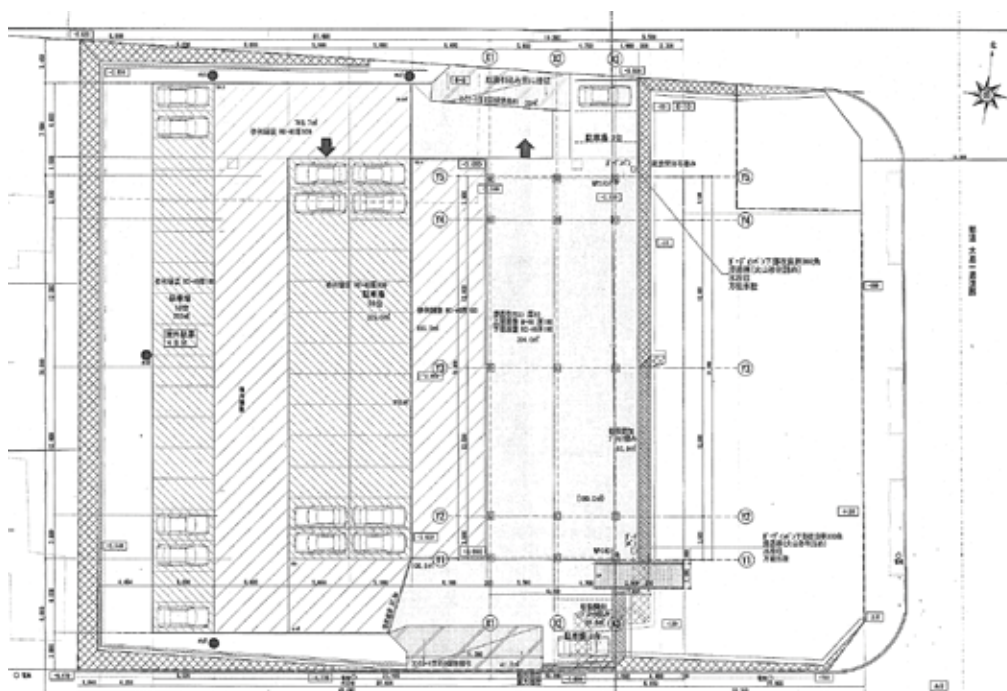
1階図面
