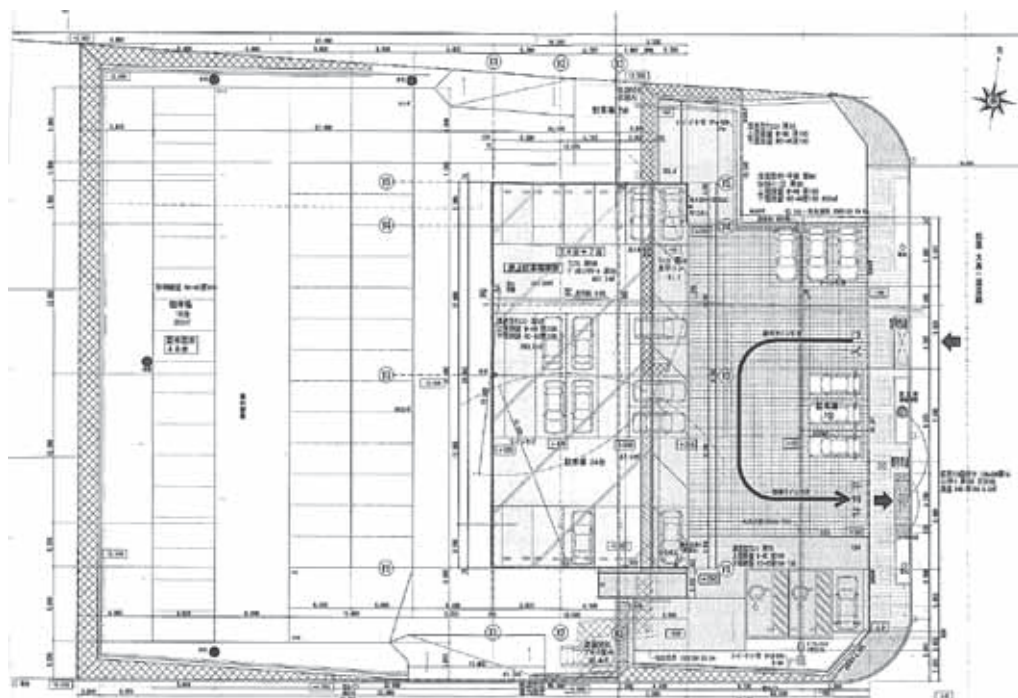
2階図面
